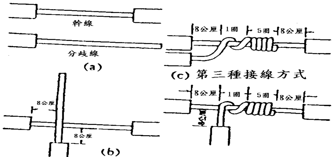
線徑2.6公厘以下(受張力)之分歧接續
