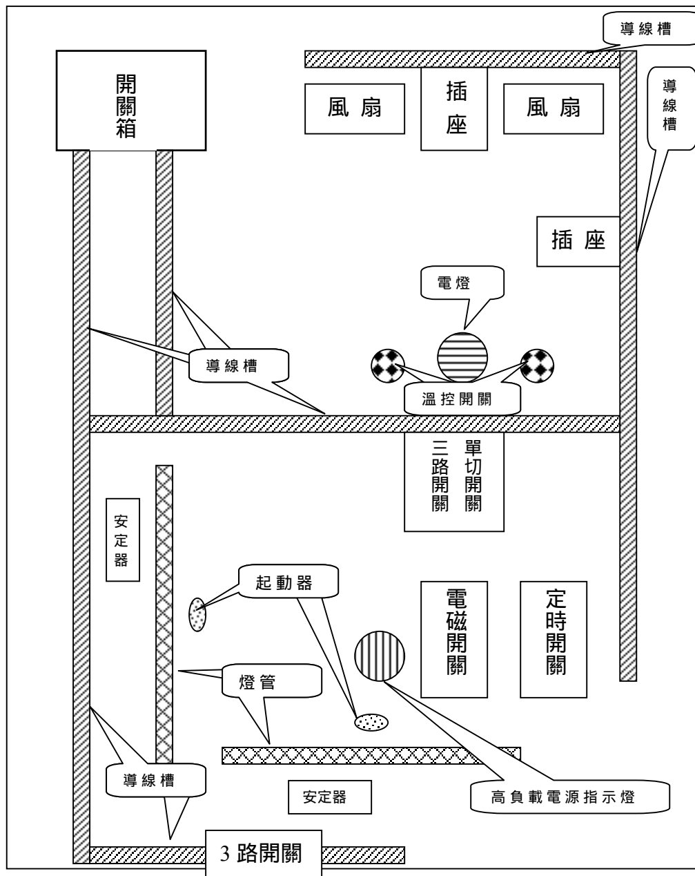
實習設備配置圖
