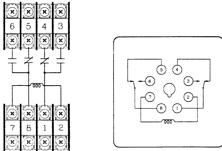
電力電驛内部接線圖(MK-2P)
