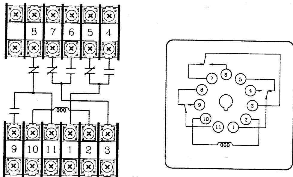
電力電驛内部接線圖(MK-3P)
