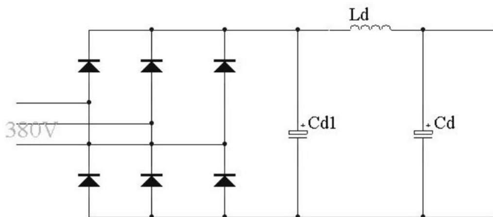
图 3.5 无源功率因数校正的电路
