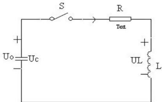
图 3.2d 主回路等效电路 4
