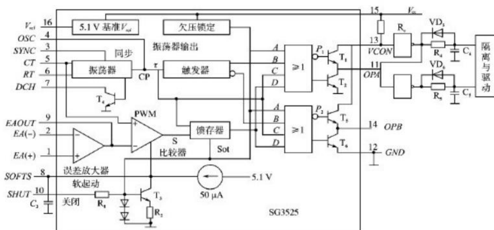
图 4.2 SG3525A 内部结构
