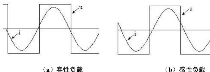
图 2.3 负载输出波形
