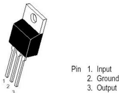
图 6.1 CW78 \times\times 、CW79 \times\times 系列稳压器
