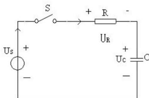
图 3.2a 主回路等效电路 1
