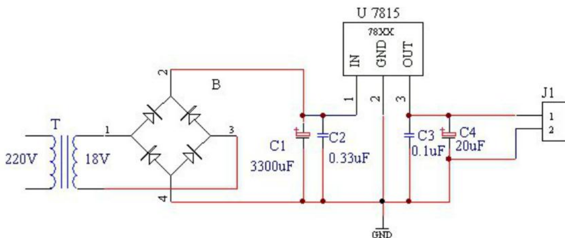
图 6.3 +15 伏稳压电压电源
