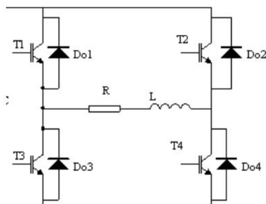
图 2.2 串联逆变器结构
